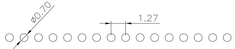
P.C.B LAYOUT
