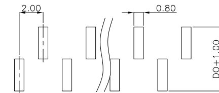
P.C.B LAYOUT
