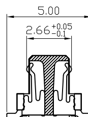
A-A SECTION
