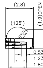
SECTION A-A SCALE 1:1
